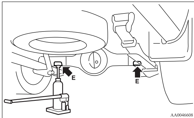
Е - Задняя точка установки домкрата
